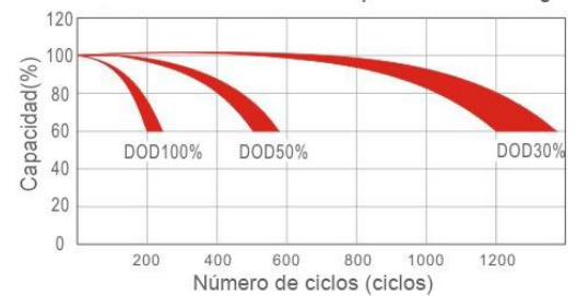
Ciclo de vida útil en relación con la profundidad de descarga
